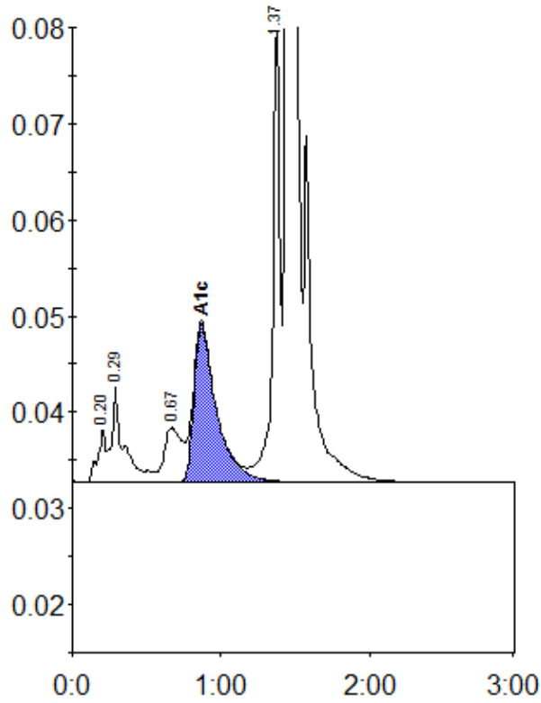
Peak table - ID: 11295397
