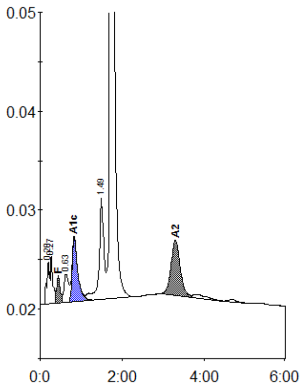
Peak table - ID: 11293477
