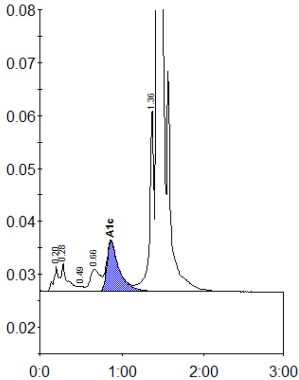
Peak table - ID: 10866410
