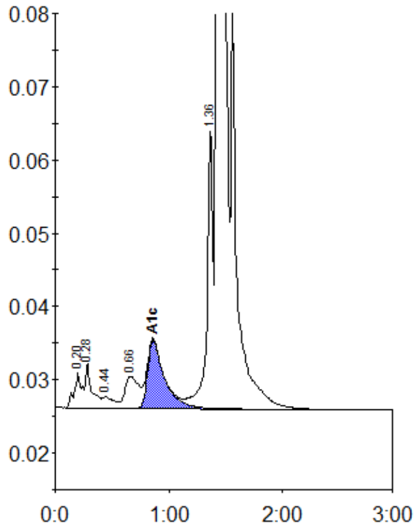
Peak table - ID: 11293779
