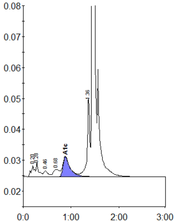
Peak table - ID: 11320977
