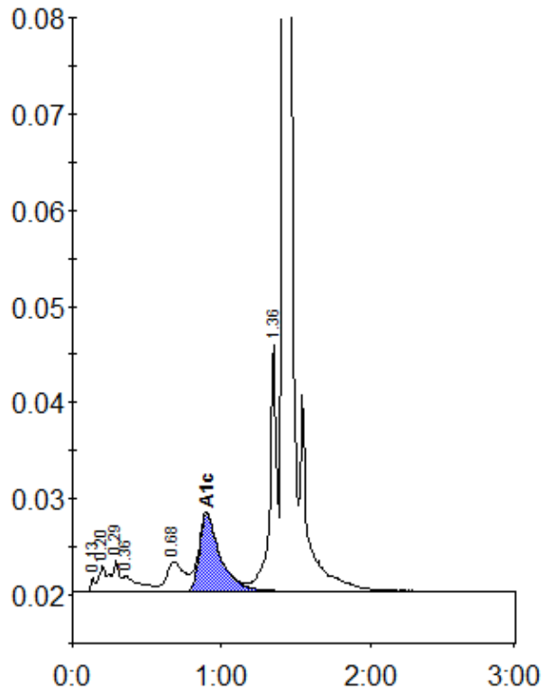
Peak table - ID: 11103446
