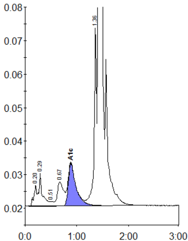
Peak table - ID: 11193594
