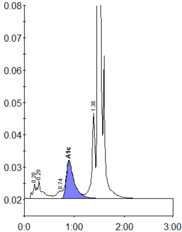
Peak table - ID: 10891555
