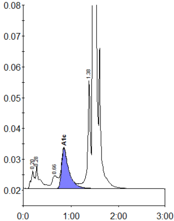
Peak table - ID: 10957234
