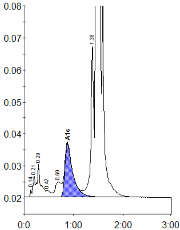
Peak table - ID: 10971564
