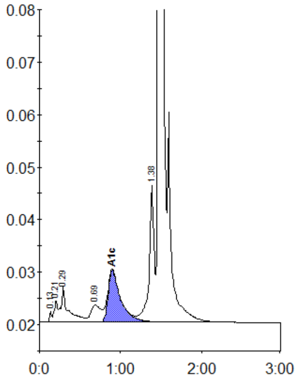
Peak table - ID: 10993508
