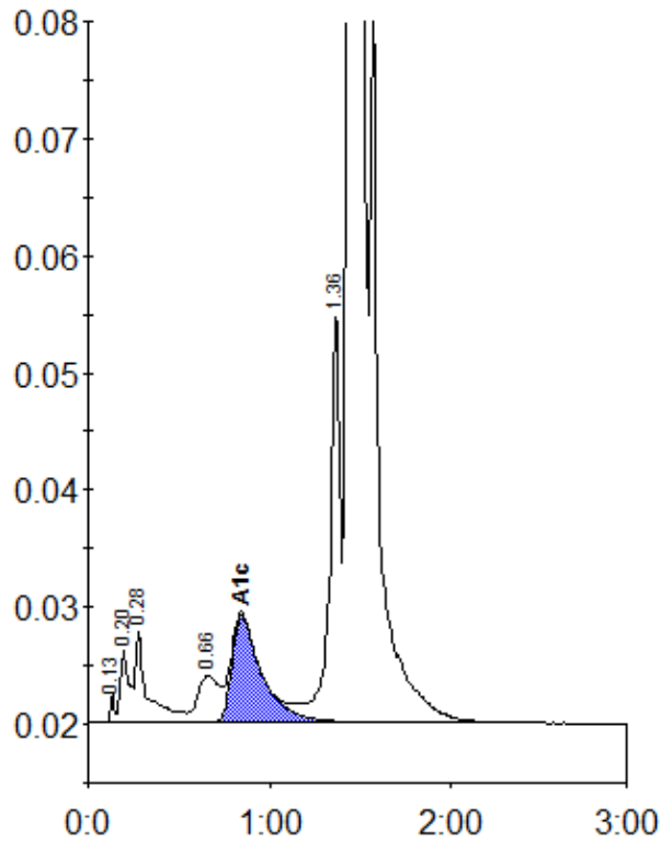
Peak table - ID: 10948331
