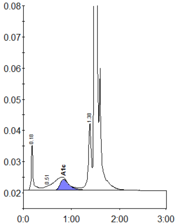
Peak table - ID: 10893104
