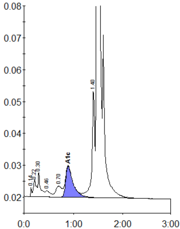
Peak table - ID: 10870199
