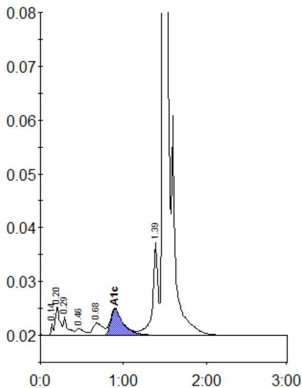
Peak table - ID: 10929599
