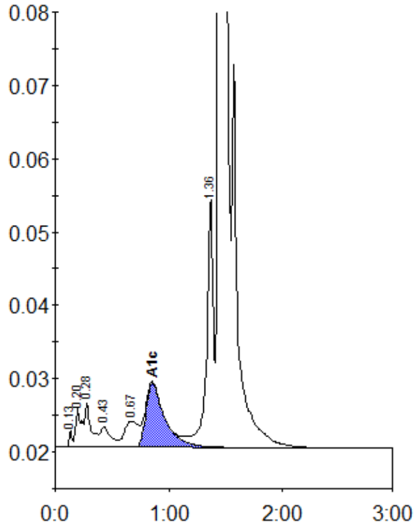
Peak table - ID: 10925348
