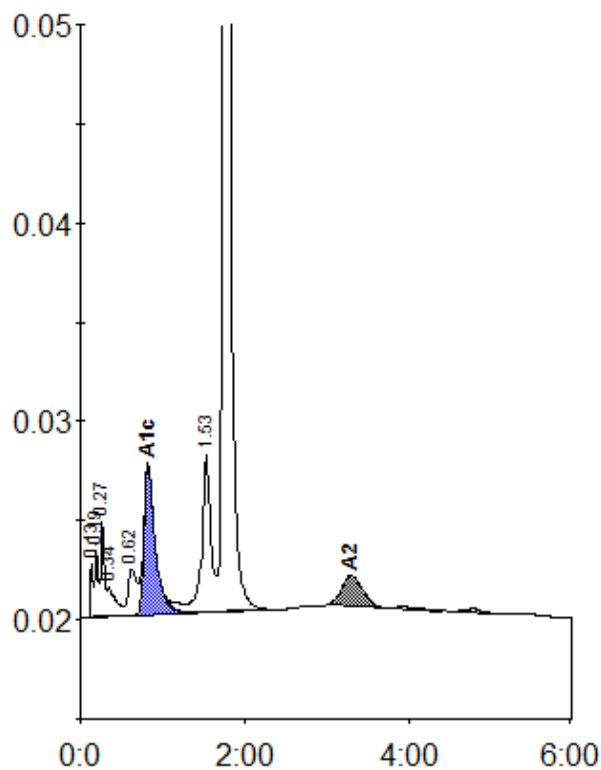
Peak table - ID: 10917917
