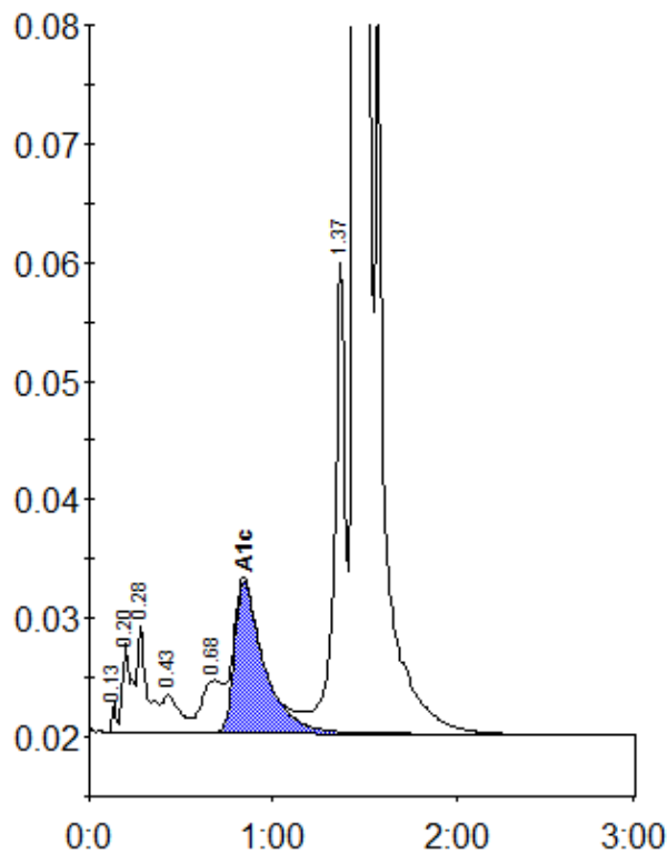
Peak table - ID: DPLTA00426500
