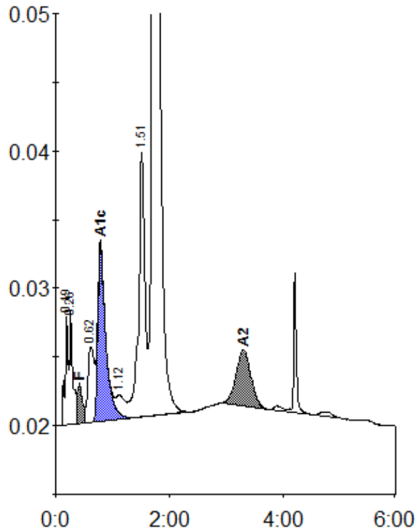
Peak table - ID: 10877808
