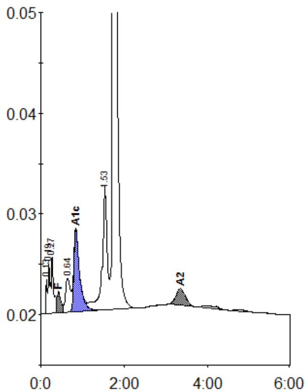
Peak table - ID: 10929534
