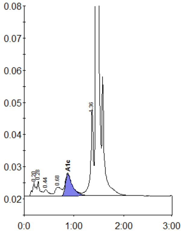
Peak table - ID: 10874724
