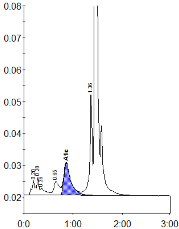
Peak table - ID: 10893773
