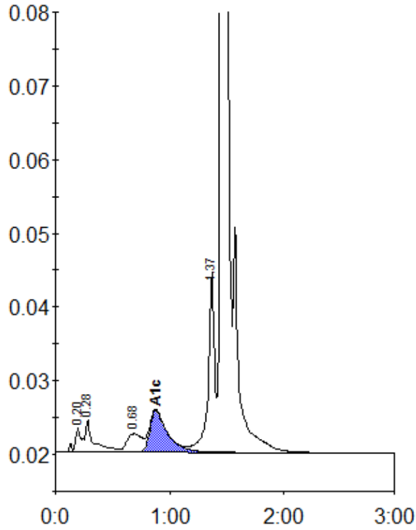
Peak table - ID: 10845581
