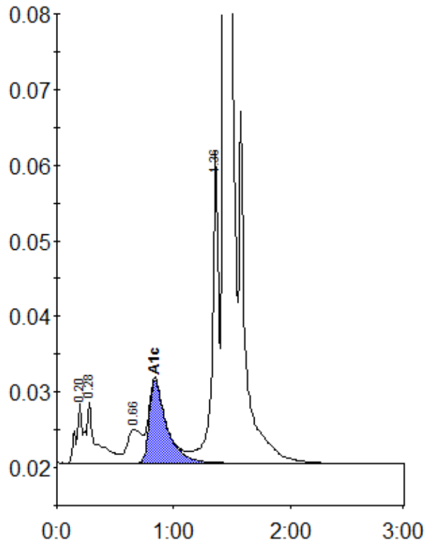
Peak table - ID: 10883974
