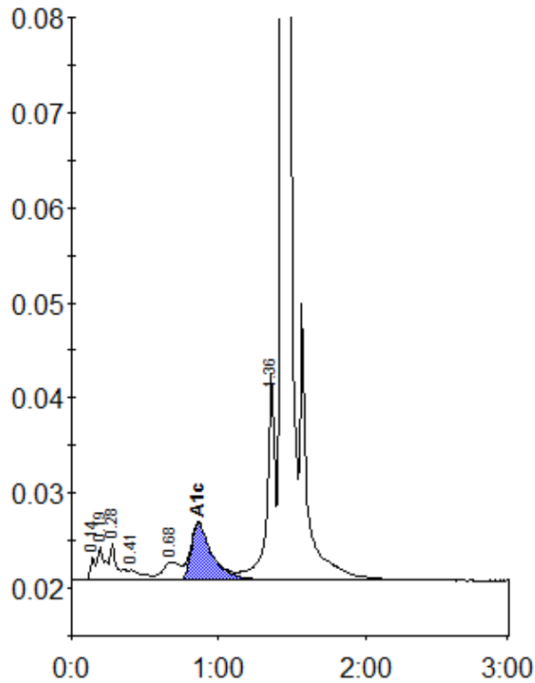
Peak table - ID: 10875491
