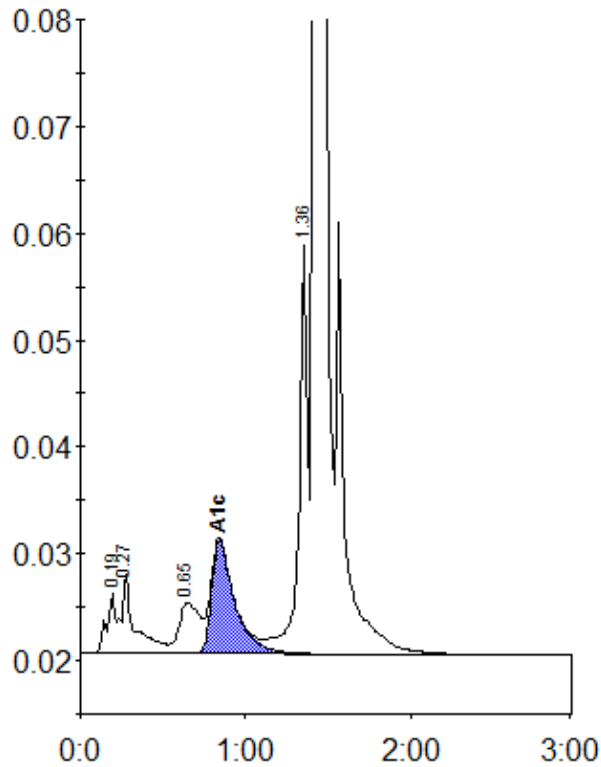
Peak table - ID: 10879897
