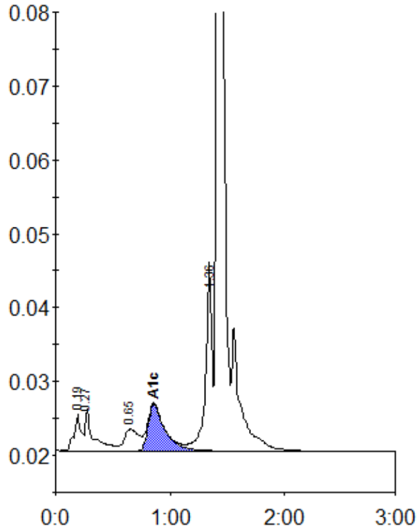
Peak table - ID: 10881592
