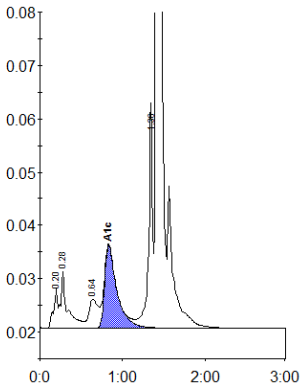
Peak table - ID: 10833789
