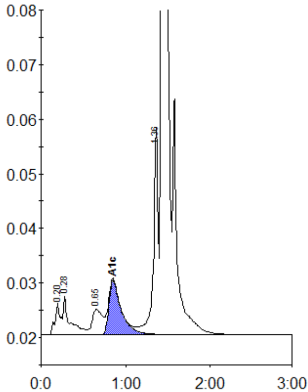
Peak table - ID: 10730356
