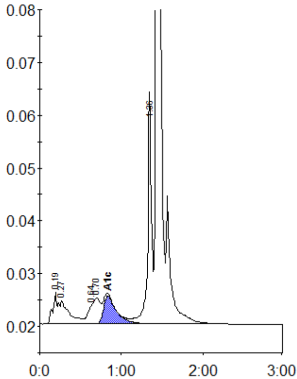
Peak table - ID: 10754240
