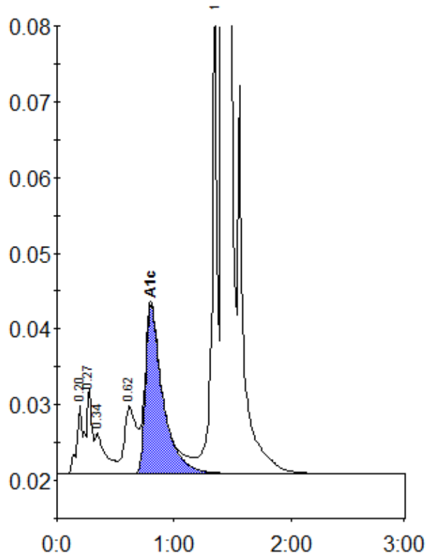
Peak table - ID: 10811822
