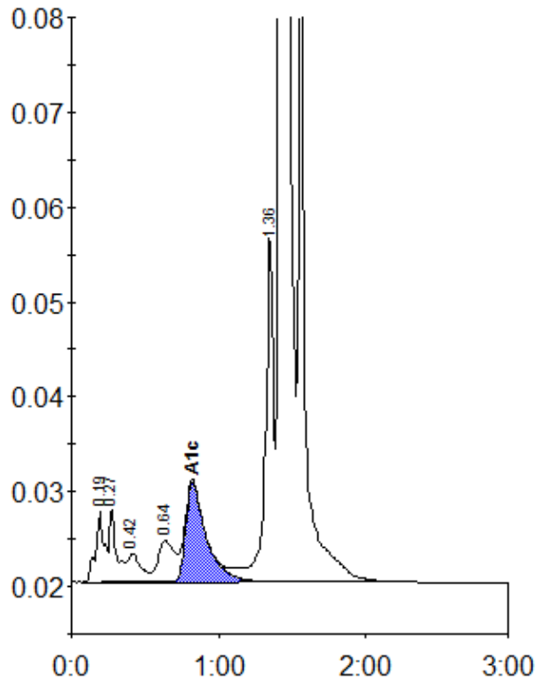
Peak table - ID: 10764166
