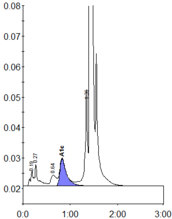
Peak table - ID: 10697420
