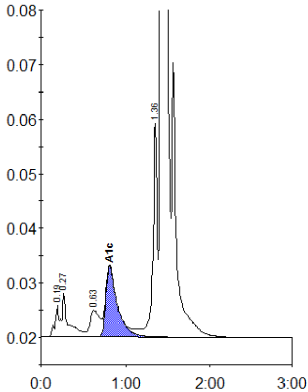
Peak table - ID: 10738947
