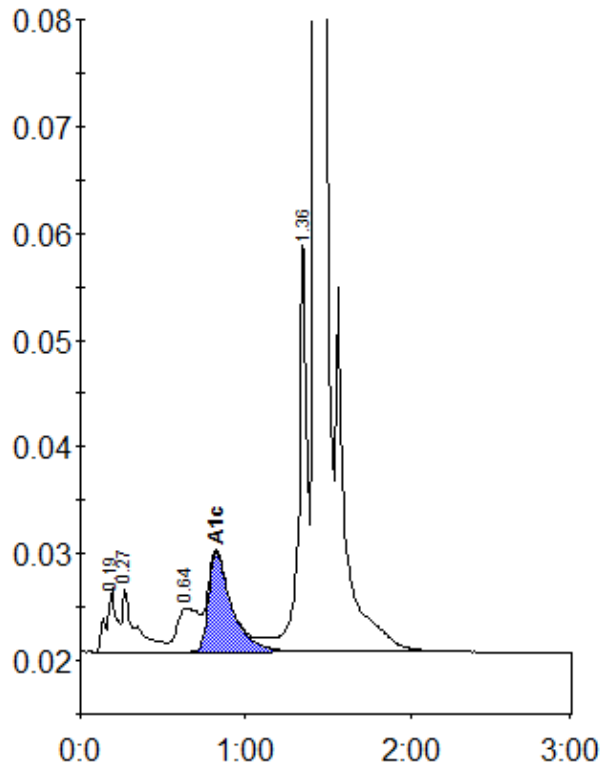
Peak table - ID: 10738492
