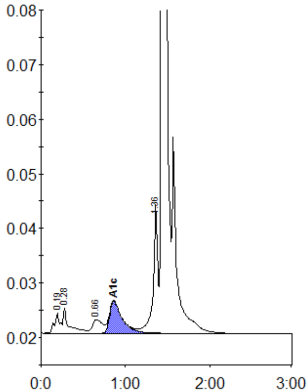
Peak table - ID: 10726384
