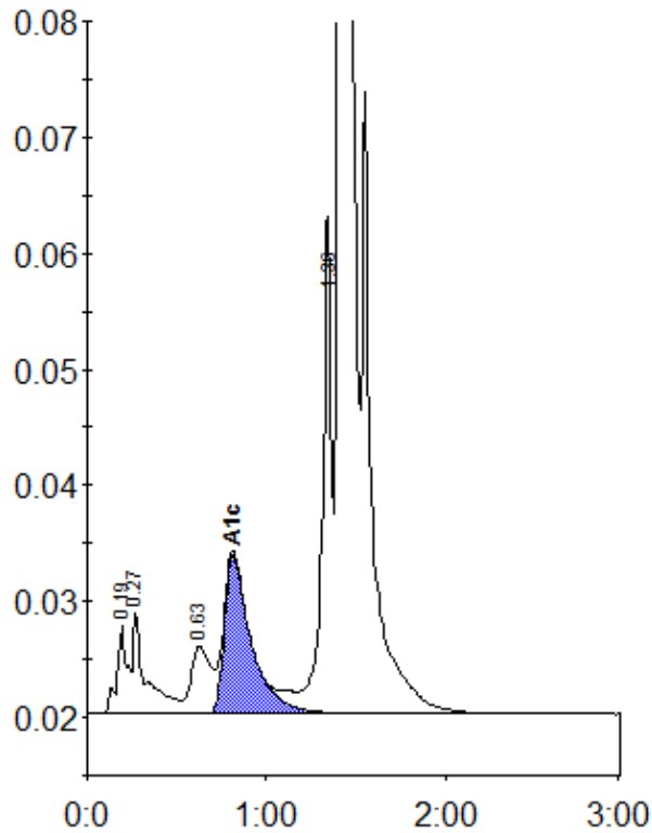
Peak table - ID: 10769343
