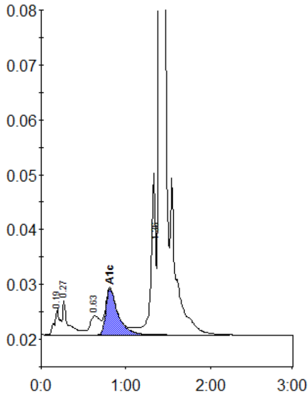
Peak table - ID: 10679496
