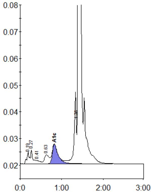
Peak table - ID: 10679497
