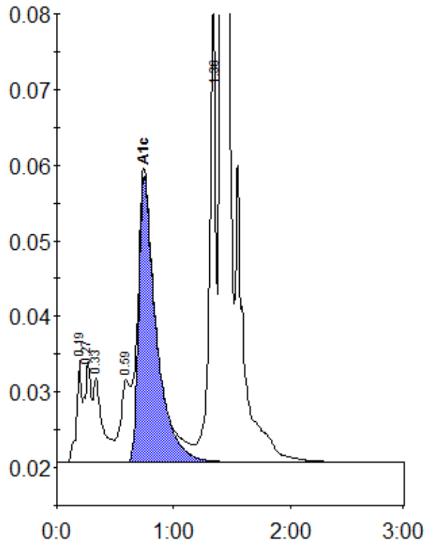
Peak table - ID: 10739923
