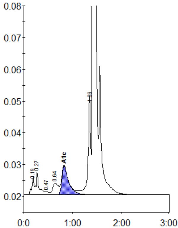
Peak table - ID: 10686735
