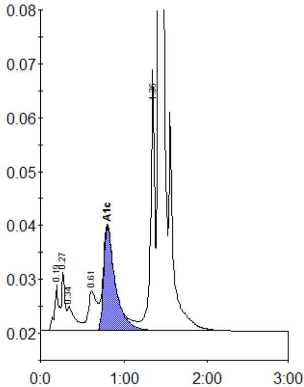
Peak table - ID: 10727238
