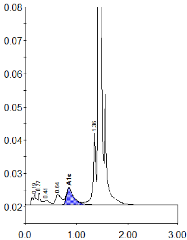
Peak table - ID: 10638415
