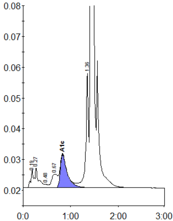
Peak table - ID: DPLTA00110142
