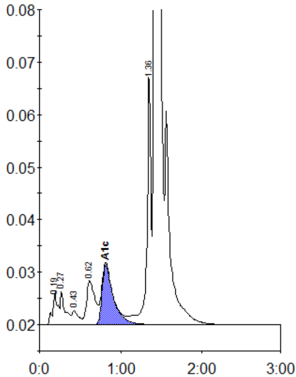
Peak table - ID: 10698881
