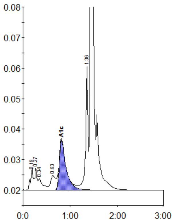
Peak table - ID: 10720457
