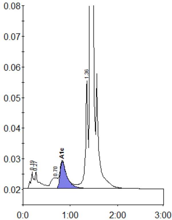
Peak table - ID: 10637216
