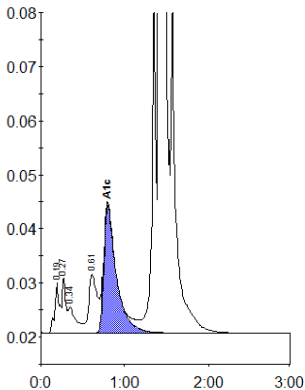
Peak table - ID: 10538955
