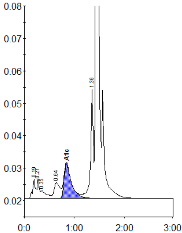
Peak table - ID: 10720860
