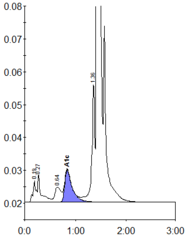
Peak table - ID: 10638763
